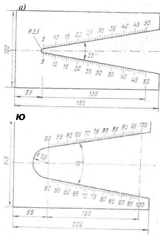
Рис. 1.10.5. Гололедный шаблон для измерения отложений.
