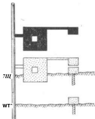
Рис. 17.3. Фотометрическое сравнение яркости нижнего изображения флажка и верхнего изображения щита при наблюдениях комплексным методом.
