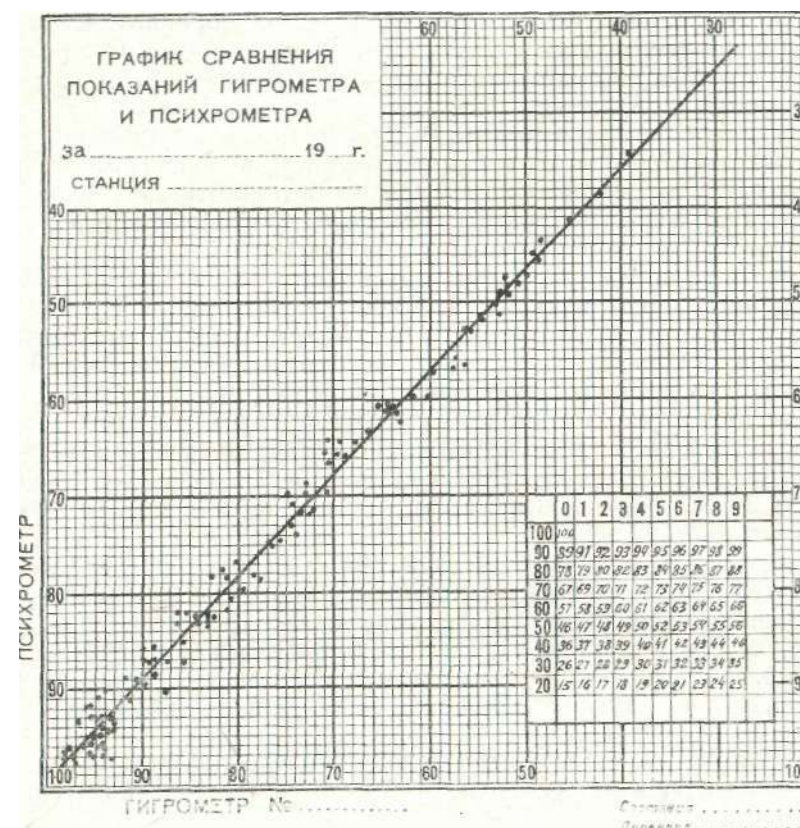
Рис. 6.2. График сравнения показаний гигрометра и психрометра.
