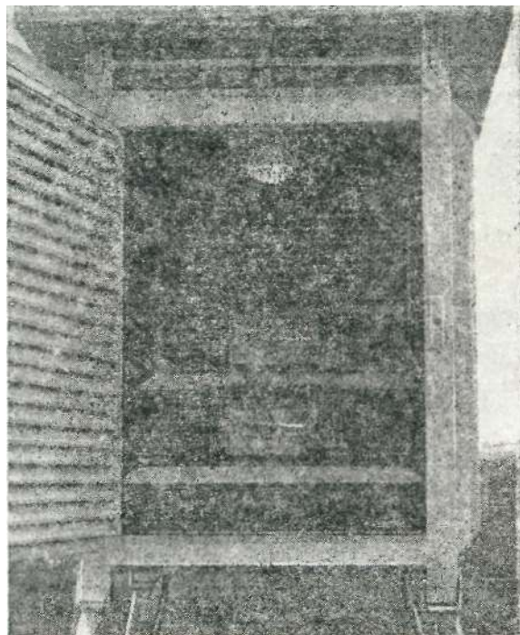
Рис. 1.5.3. Размещение термографа и гигрографа в защитной будке типа БС.
