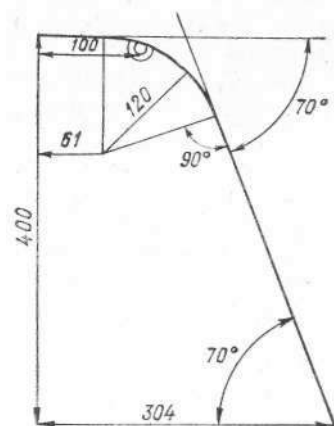
Рис. 1.8.2. Шаблон для проверки изгиба пластинок к осадкомеру.
