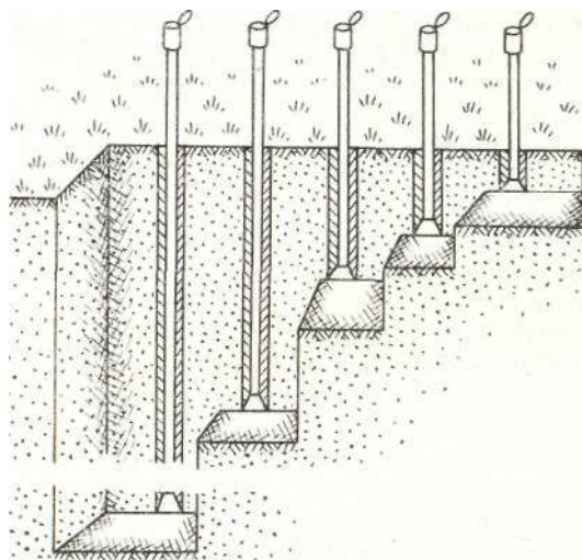
Рис. 1.7.6. Установка вытяжных почвенно-глубинных термометров.
