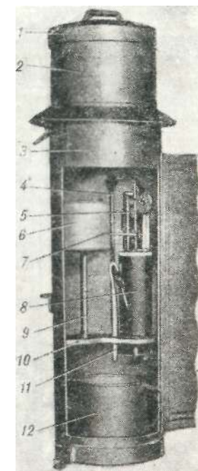
Рис. 1.8.3. Измерительный стакан осадкомера.
