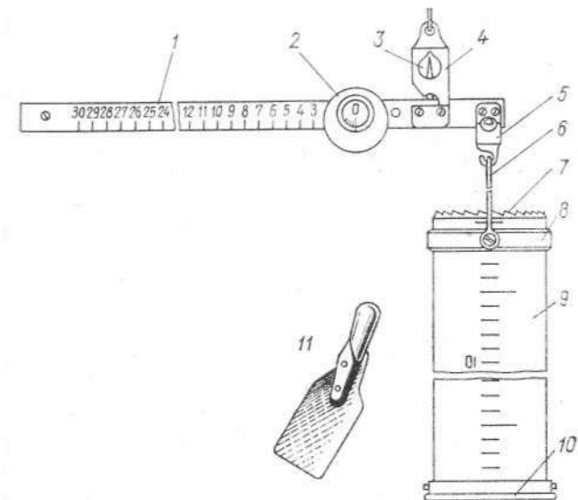
Рис. 1.9.2. Снегомер весовой ВС-43.
