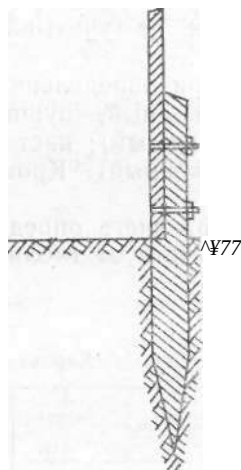
Рис. 13.1. Крепление постоянной снегомерной рейки.
