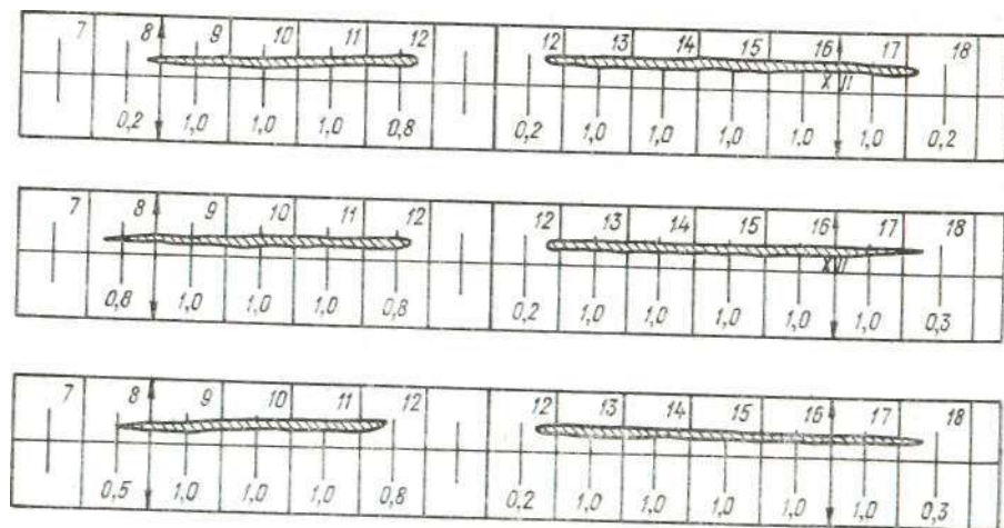
Рис. 1.6.5. Запись на лентах гелиографа в случае затенения прибора при восходе и заходе солнца.
