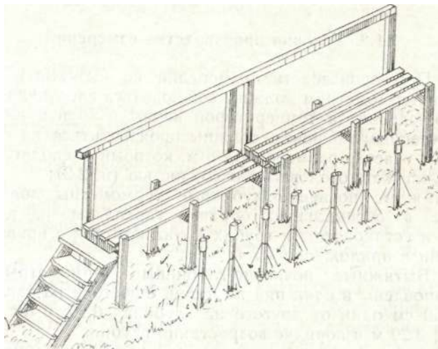
Рис. 11.1. Общий вид установки вытяжных почвенно-глубинных термометров.
