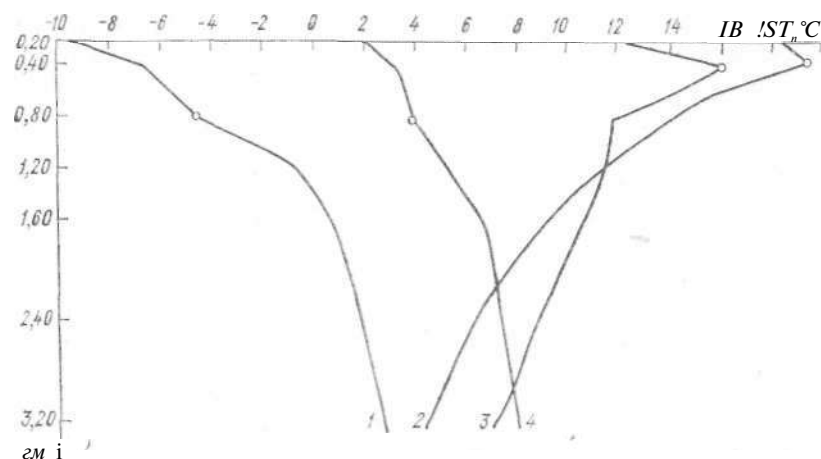
Рис. 1.7.10. Примеры неправильного распределения температуры почвы на глубинах под естественным покровом.
