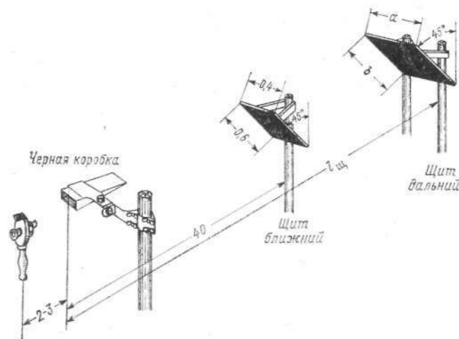
Рис. 1.12.1. Схема размещения оборудования при наблюдениях по методу фотометрического сравнения.
