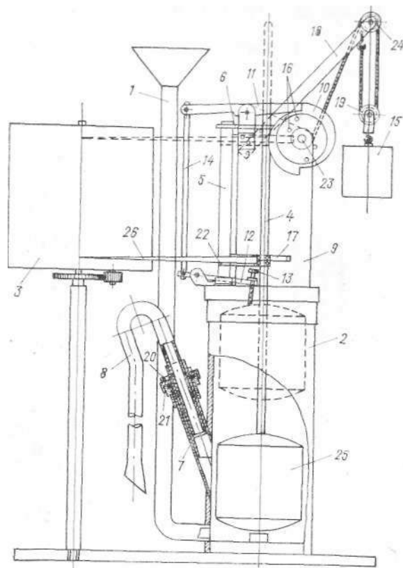
Рис. 1.8.5. Механизм принудительного слива плювиографа.
