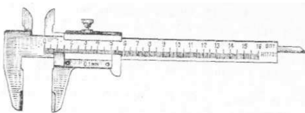
Рис. 1.10.4. Штангенциркуль.
