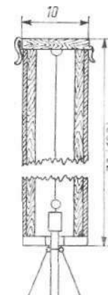
Рис. 1.7.8. Деревянный футляр для защиты вытяжных почвенно-глубинных термометров при высоком снежном покрове (разрез).
