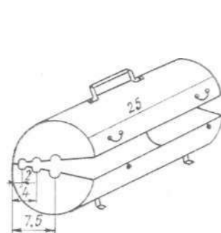
Рис. 1.10.2. Ванна для оттаивания гололедного отложения.
