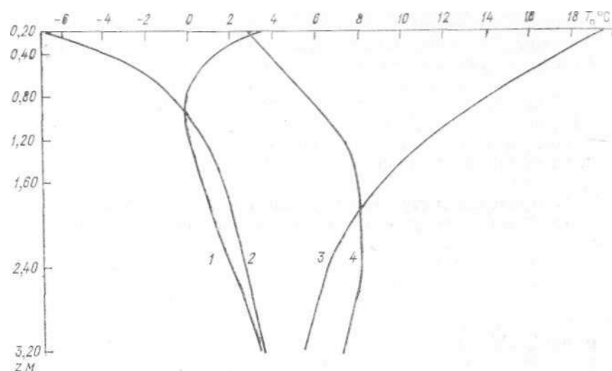
Рис. 1.7.9. Примеры правильного распределения температуры почвы на глубинах под естественным покровом.
