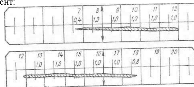
Рис. 1.6.3. Запись на ленте гелиографа при нарушении горизонтальности установки прибора по линии запад—восток.
