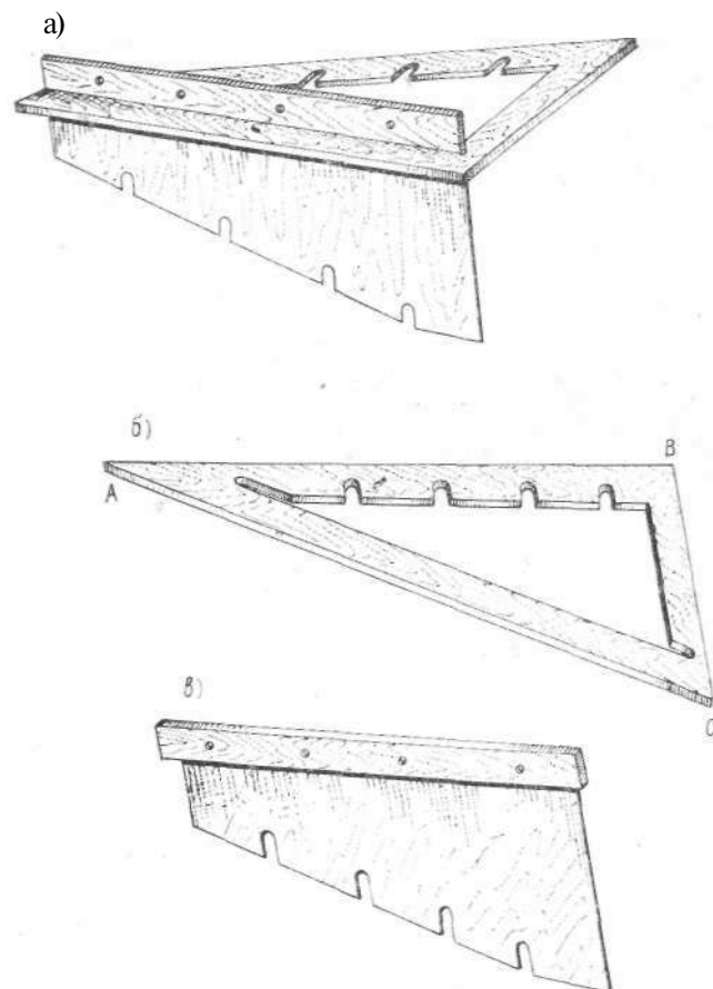
Рис. 1.7.4. Шаблон для установки коленчатых термометров.
