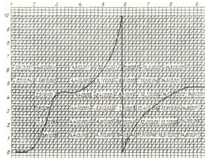
Рис. 12.1. Образец обработанного бланка плювиографа?
