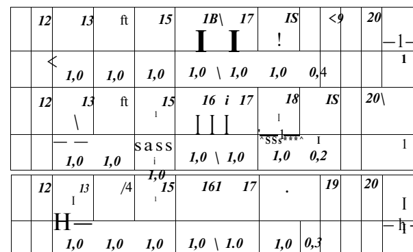
Рис. 1.6.6. Запись на лентах гелиографа при затенении прибора в промежутке 16—17%.
