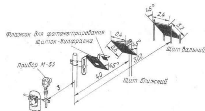
Рис. 1.12.3. Схема размещения оборудования при наблюдениях по комплексному способу.
