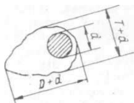
Рис. 15.1. Схема измерения диаметра и толщины отложения.
