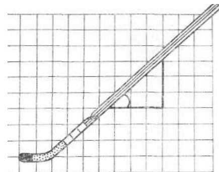
Рис. 1.7.2. Нанесение кольцевой метки на оболочку коленчатого термометра.
