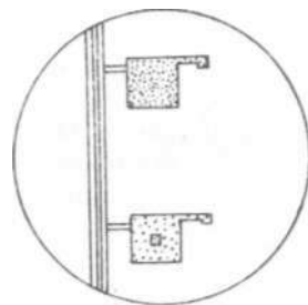
Рис. 17.4. Гашение контраста щитка-диафрагмы и дальнего щита при наблюдениях методом относительной яркости.
