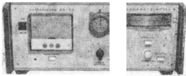
Рис. 1.3.1. Анеморумбометр М-63М-1.
