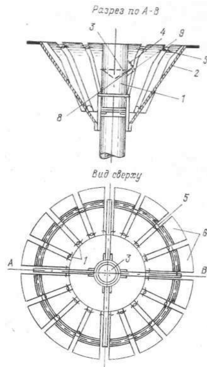
Рис. 1.8.2. Шаблон для проверки изгиба пластинок к осадкомеру.
