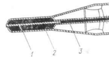
Рис. 1.4.3. Резервуар максимального термометра.
