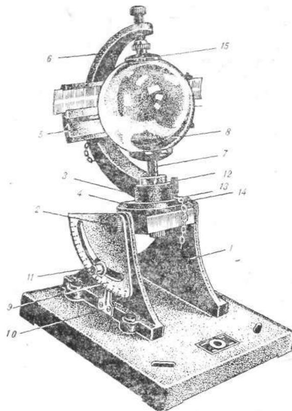
Рис. 1.6.1. Гелиограф универсальный модели ГУ-1.
