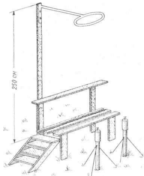
Рис. 1.7.7. Реечный помост и кольцо для опоры при производстве отсчетов по термометрам.
