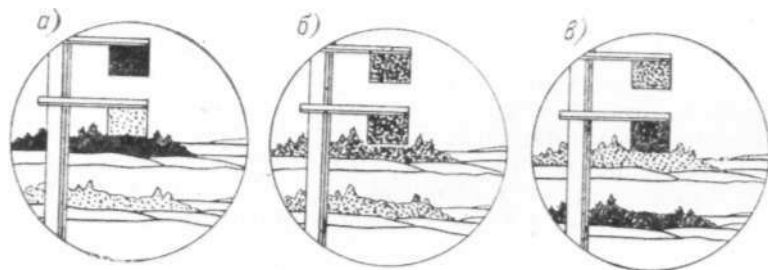
Рис. 17.2. Последовательные стадии наблюдений по методу фотометрического сравнения.
